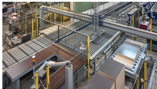
Rund 4.000 m 2 große Holzfertigung
